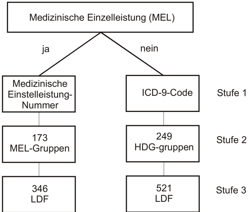
Abb. 16. LKF Baumalgorithmus
